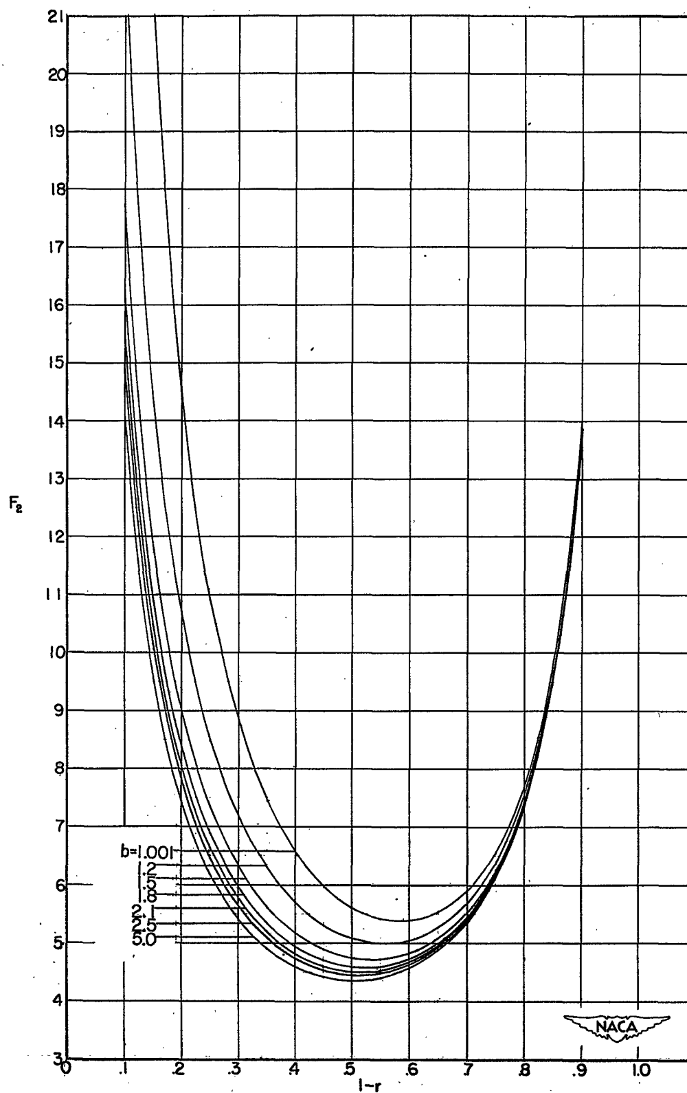
(b) F_2(r, b) .
