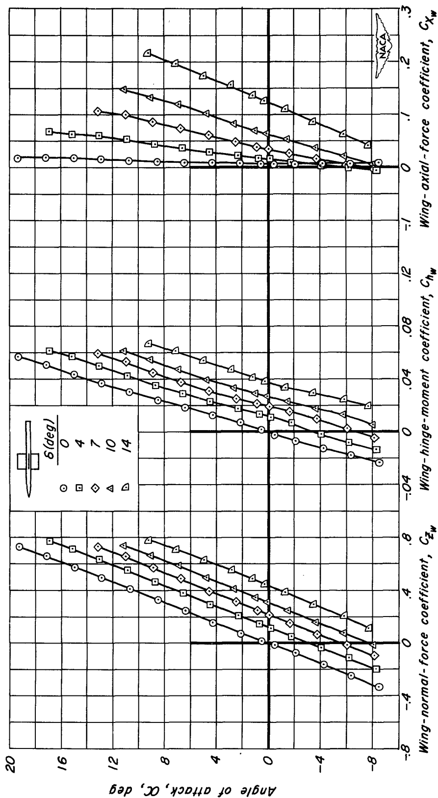
(d) Wing panel 3; Mach number, 1.9.
