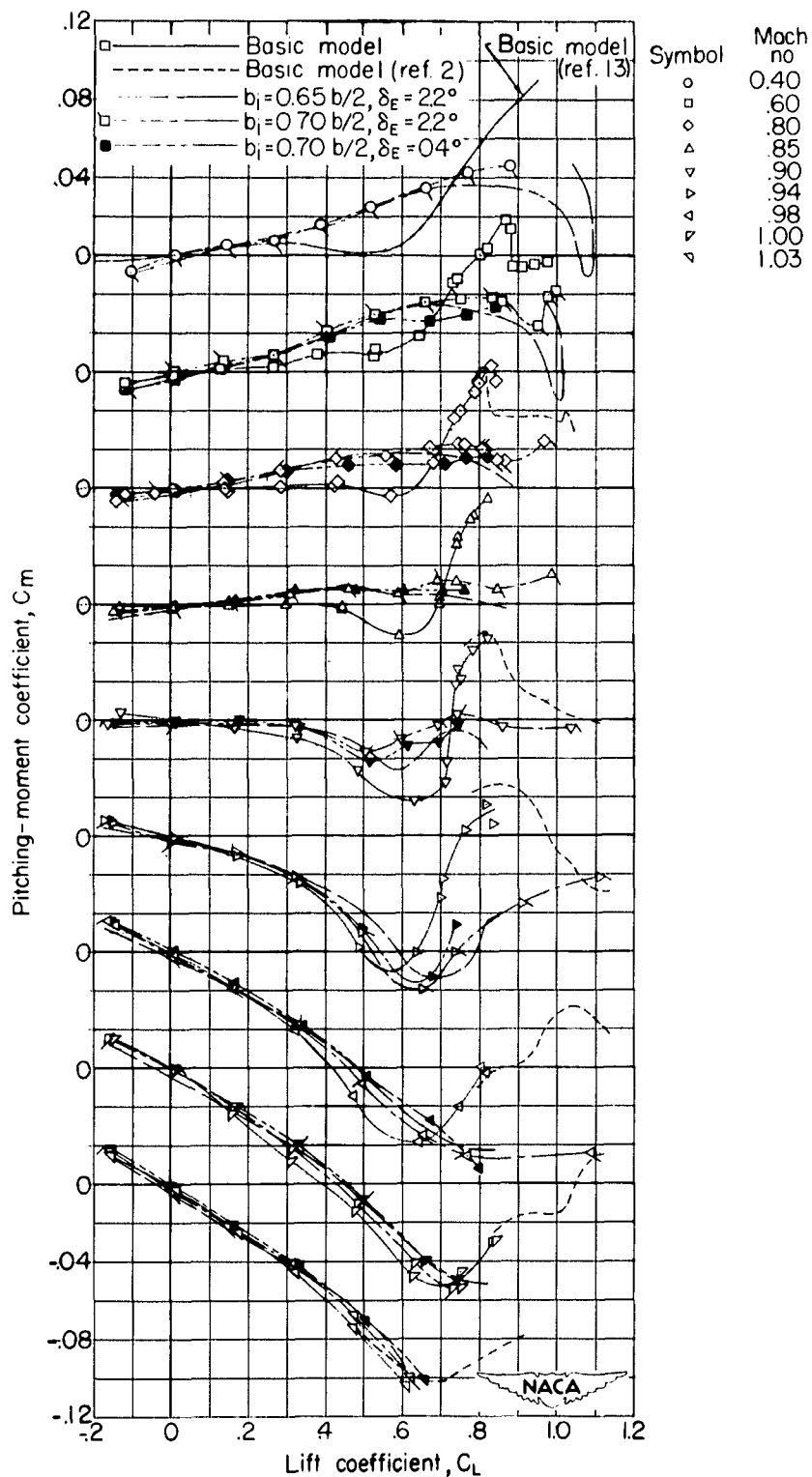
(d) Pitching moment.
