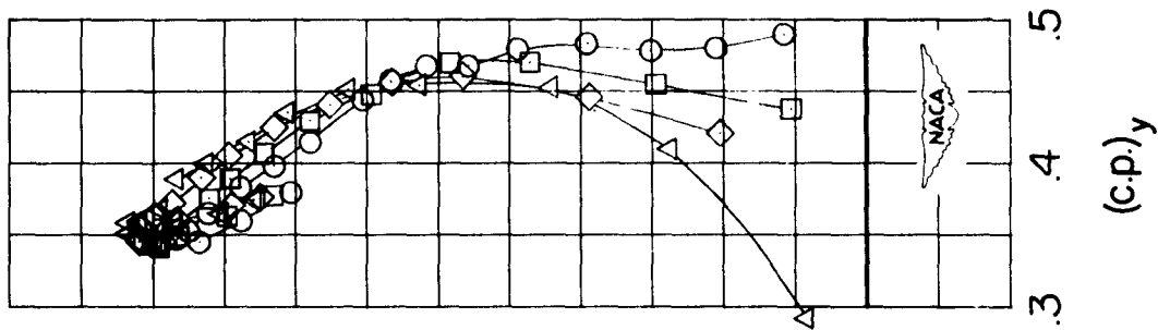
(d) C_L versus (c.p.)_y .
