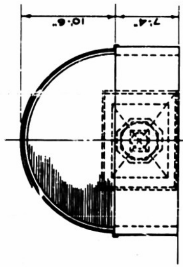
END ELEVATION
