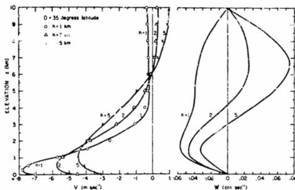
Figure 2 (a). D = 35^\circ latitude ( \equiv D_1 ).
