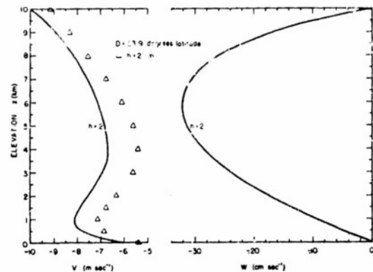
Figure 2 (b). D = 53.9^\circ latitude ( \equiv D_2 ).
