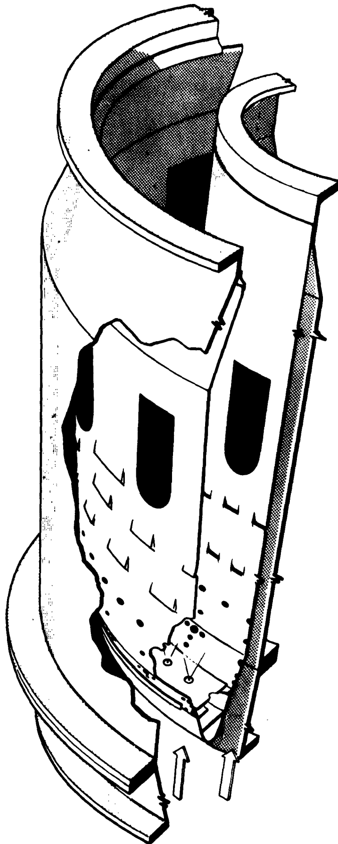
(a) Combustor A.
