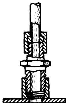
(d) Static-pressure orifice.
