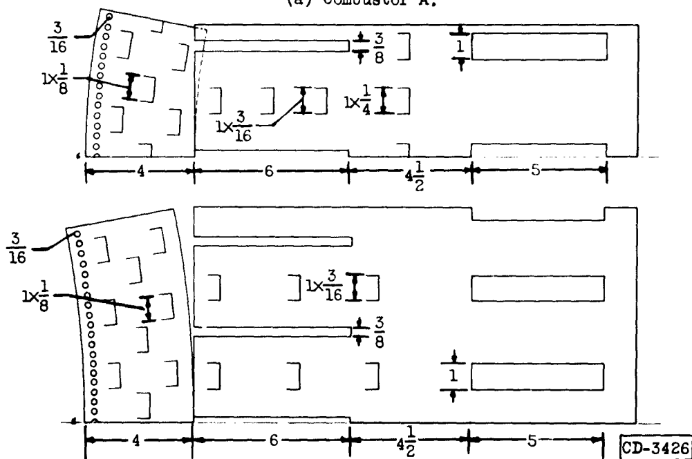
(a) Combustor A.
