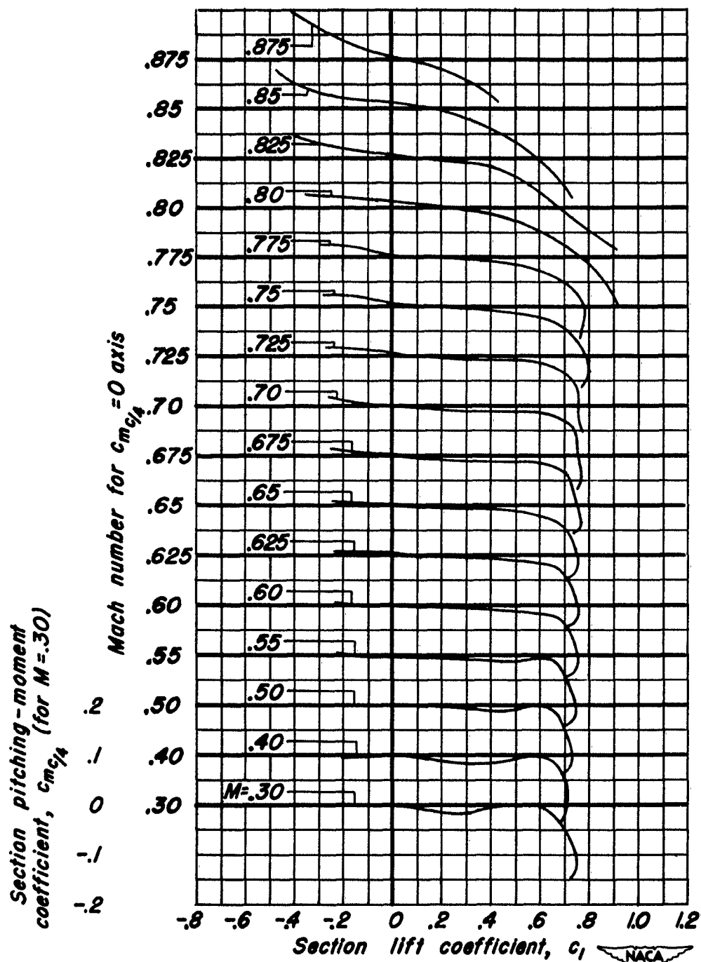
(d) NACA 0006-0.70 40/1.575 Airfoil.
