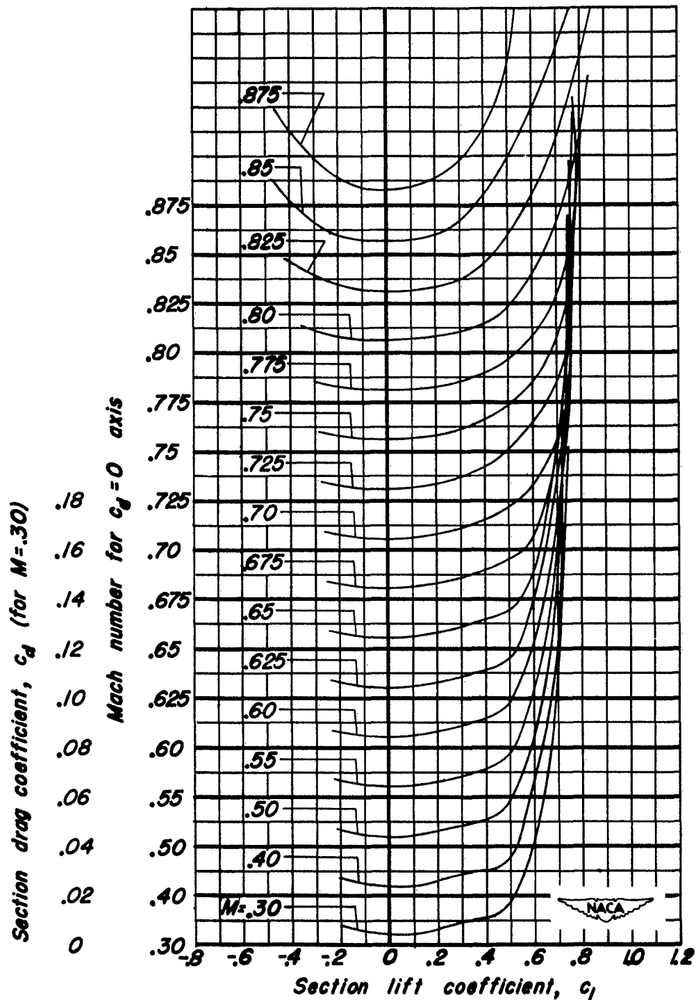
(d) NACA 0006-0.70 40/1.575 Airfoil.
