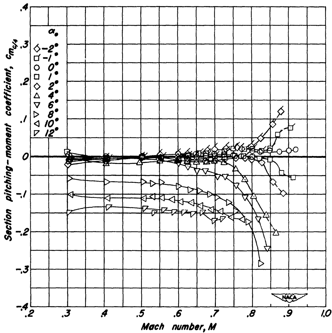
(d) NACA 0006-0.70 40/1.575 Airfoil.
