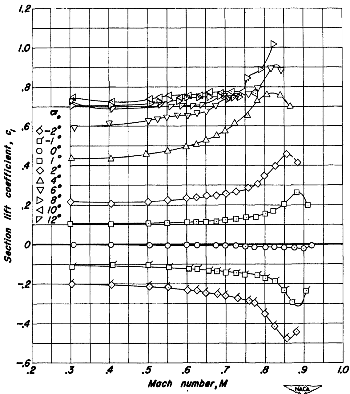
(d) NACA 0006-0.70 40/1.575 Airfoil.
