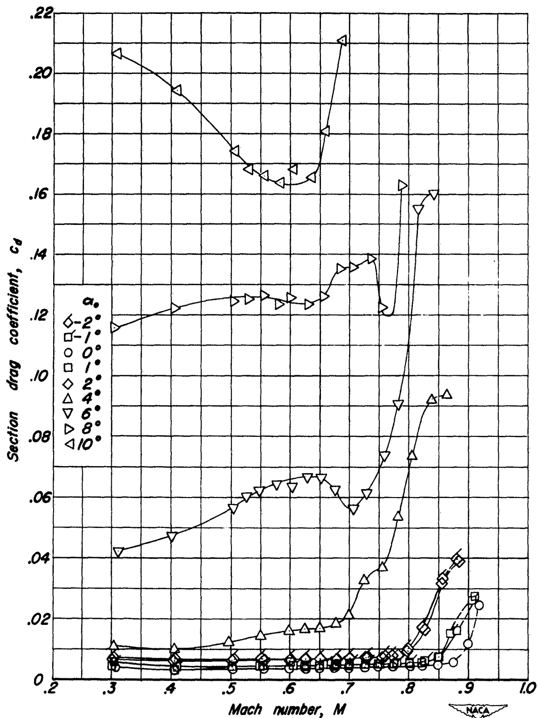
(d) NACA 0006-0.70 40/1.575 Airfoil.
