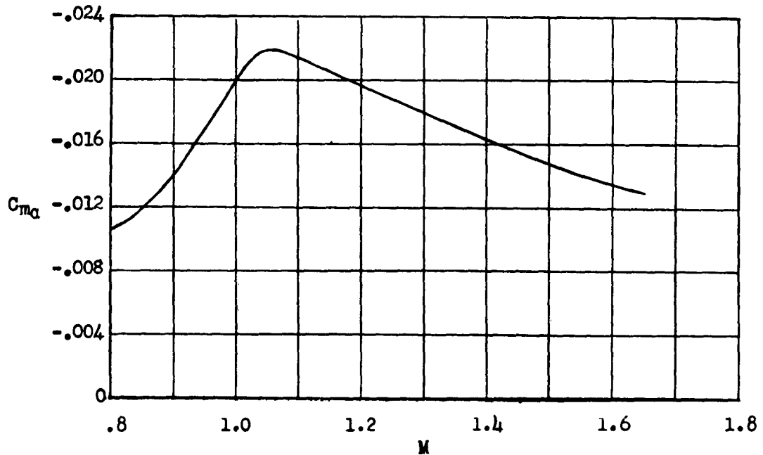
Figure 14.- Static longitudinal-stability parameter C_{m\alpha} .
