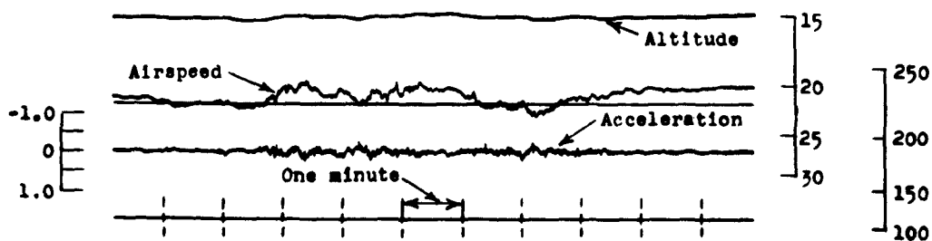
(d) Combination of maneuver and gust accelerations.
