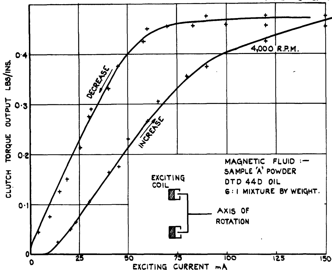
FIG. 6. TORQUE HYSTERESIS.
