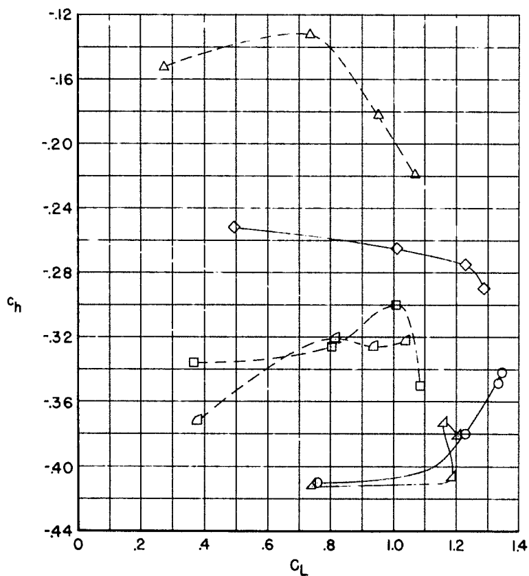
(d) c_h against C_L .
