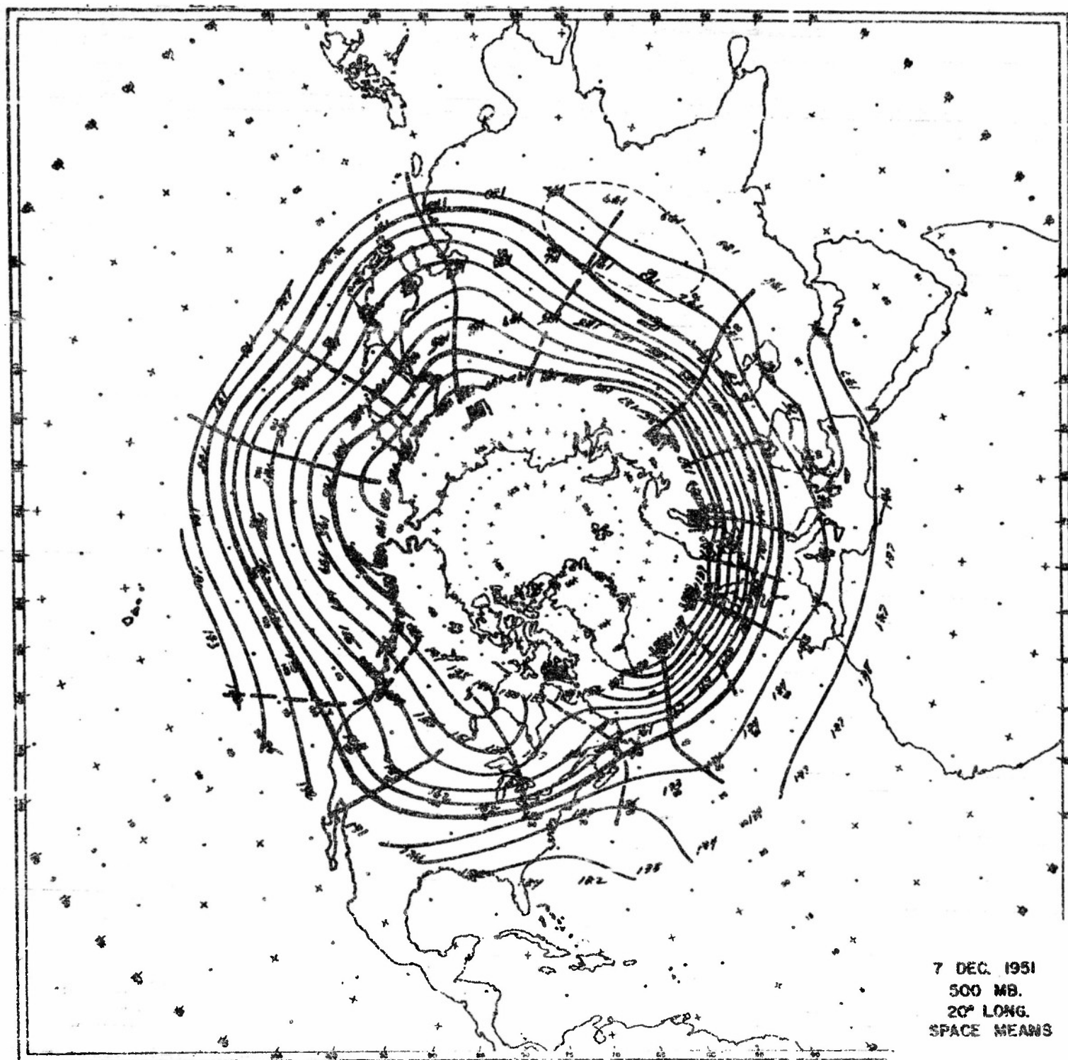
Figure (1e). Space Mean - 20° Longitude - 7 December 1951
