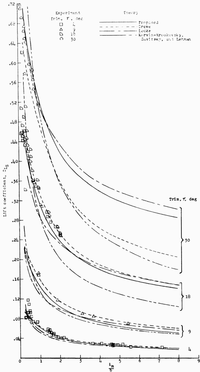
(b) Trim of 4°, 9°, 18°, and 30°.
