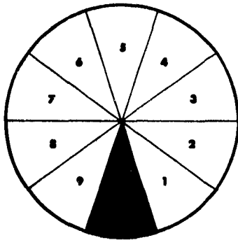
Fig. 2A 10 EQUIPROBABLE ALTERNATIVES H = 3.33
