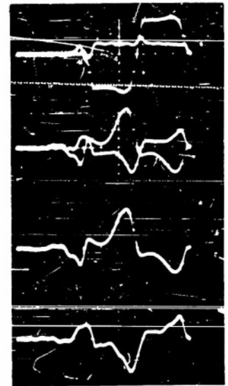
R_p = 100 R_1 = R_2 = \infty FIG. 6
