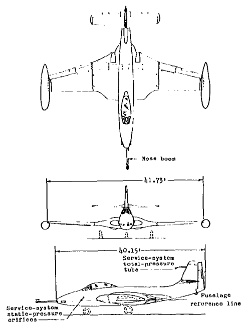
F2H-2
