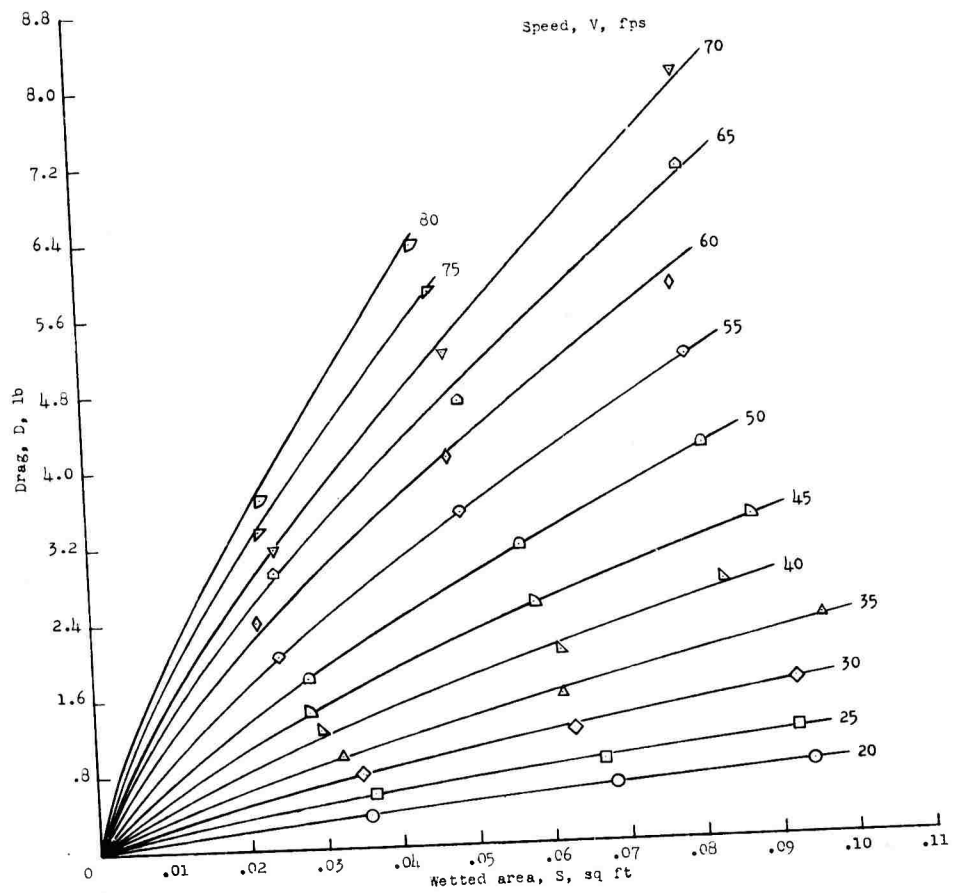
(b) Drag.
