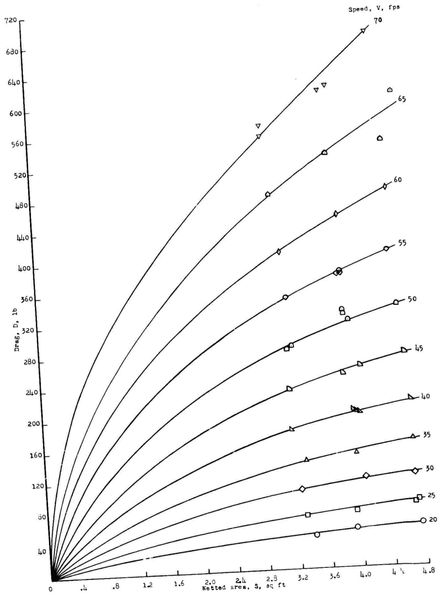
(b) Drag.
