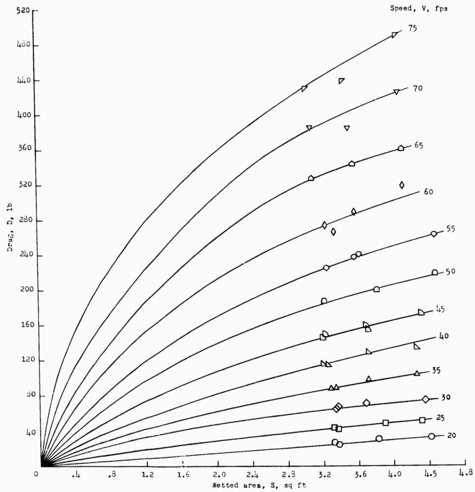
(b) Drag.
