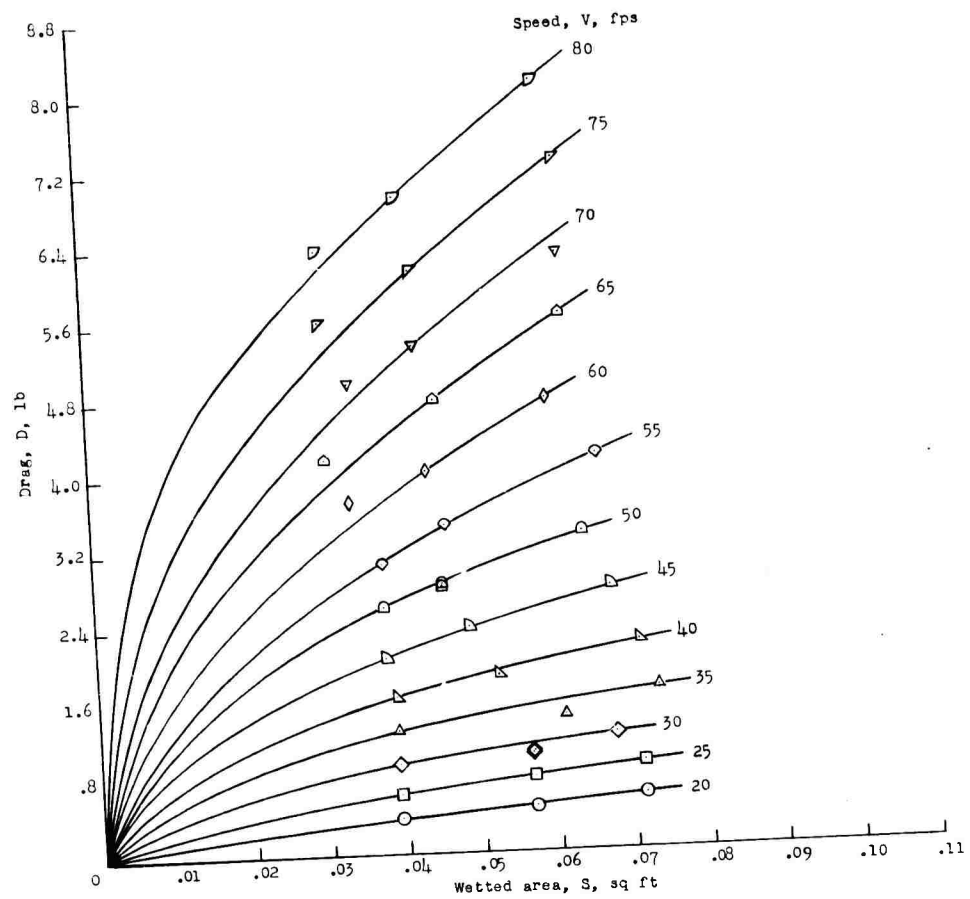
(b) Drag.
