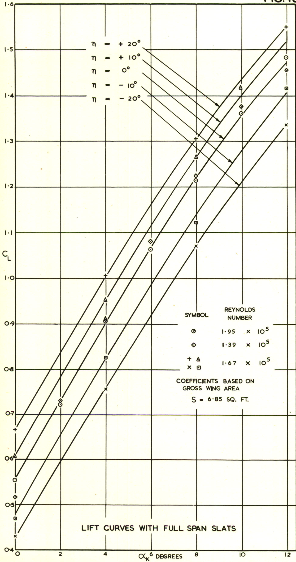
FIG.4d.
