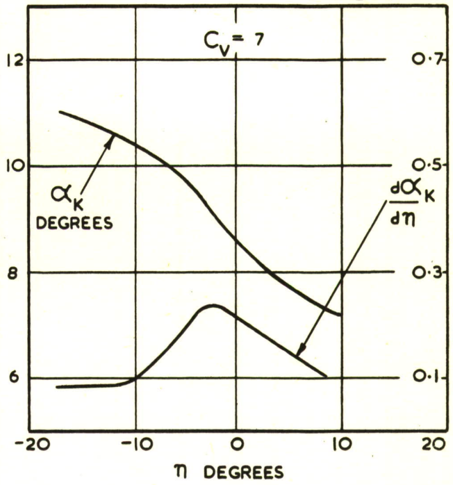
FIG. 14d.
