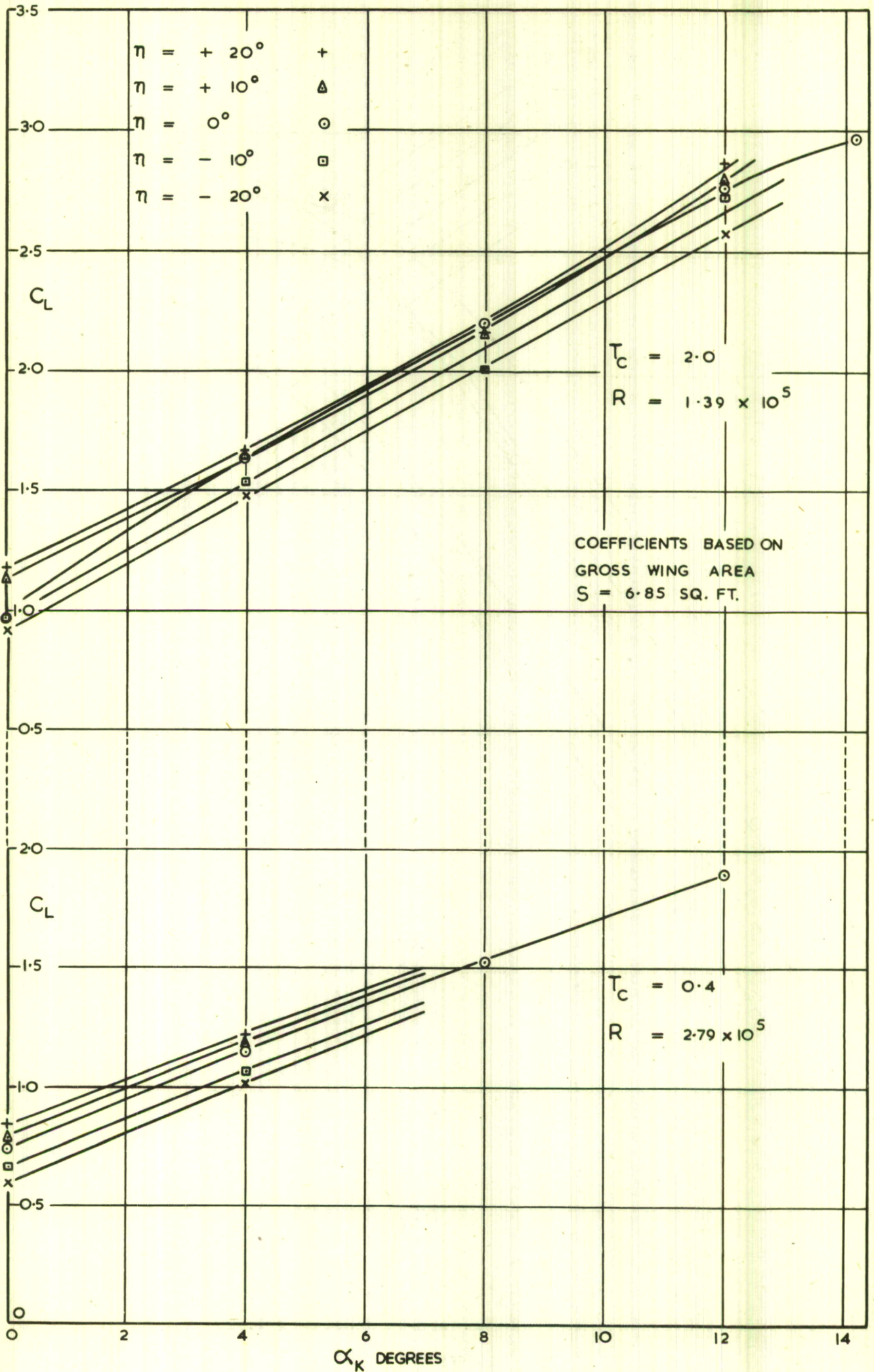
FIG. 4a.(2).
