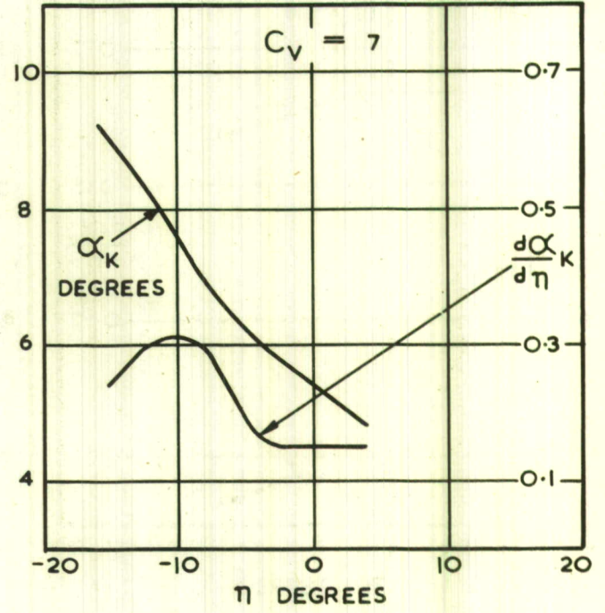
FIG.14a.
