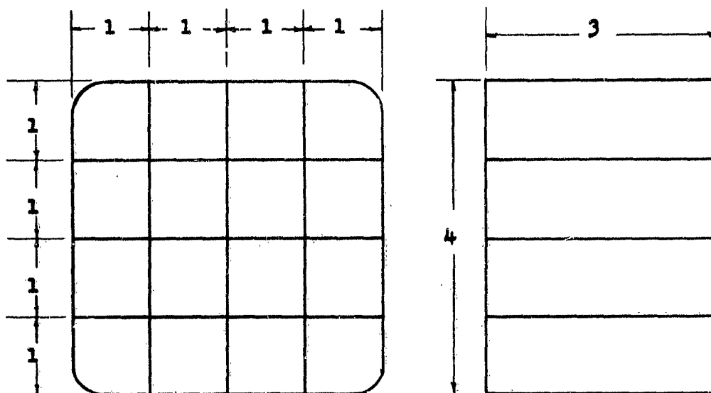
LONGITUDINAL 0.5 IN. DIA. NOTCH-TENSILE SPECIMENS
