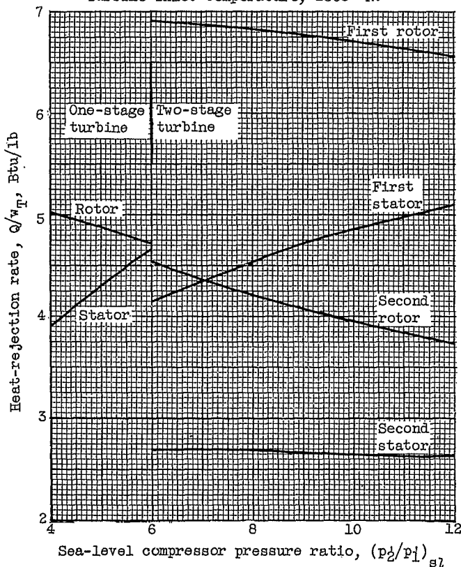
(d) Heat-rejection rate. Turbine-inlet temperature, 2800^\circ\text{R} .
