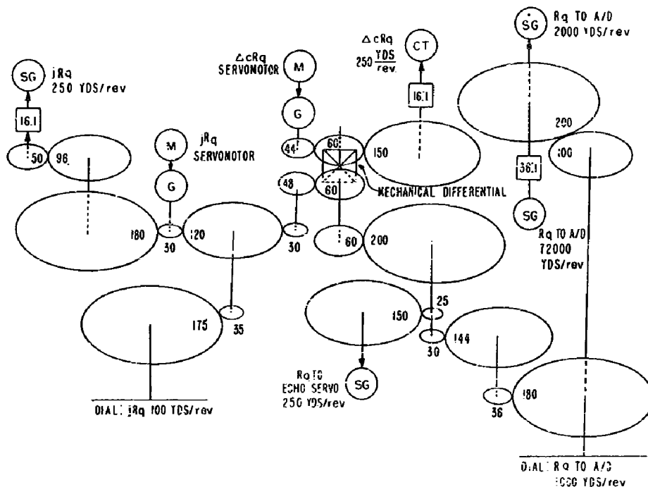
Fig. A6 - jRq and ΔcRq servos
