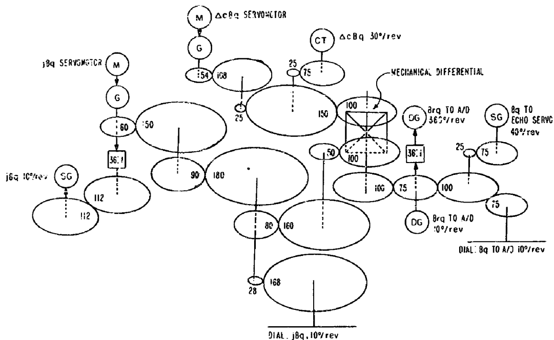
Fig. A5 - jBq and ΔcBq servos
