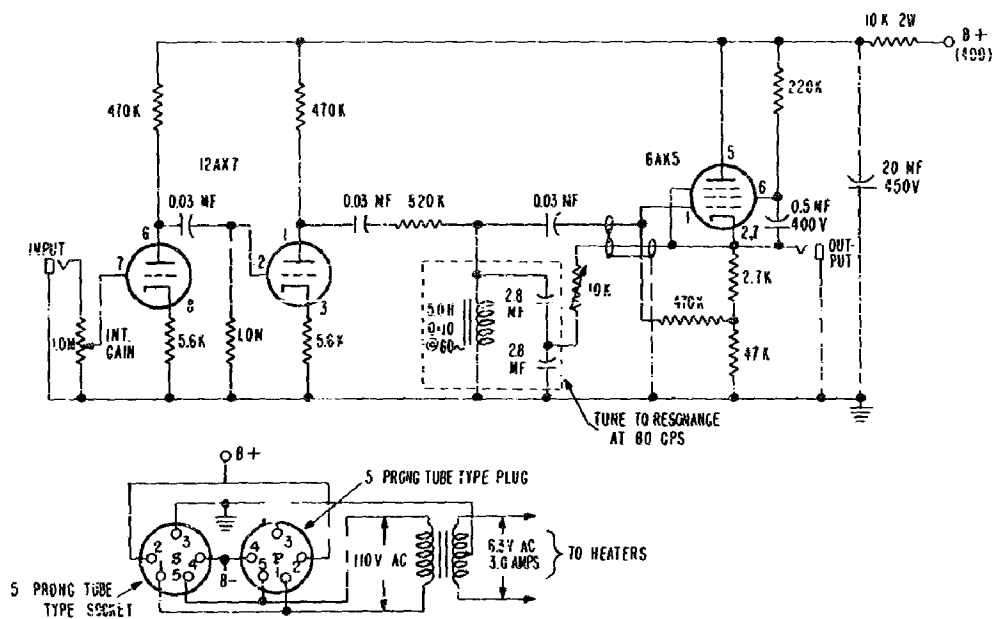
Fig. 12 - Servo integrator
