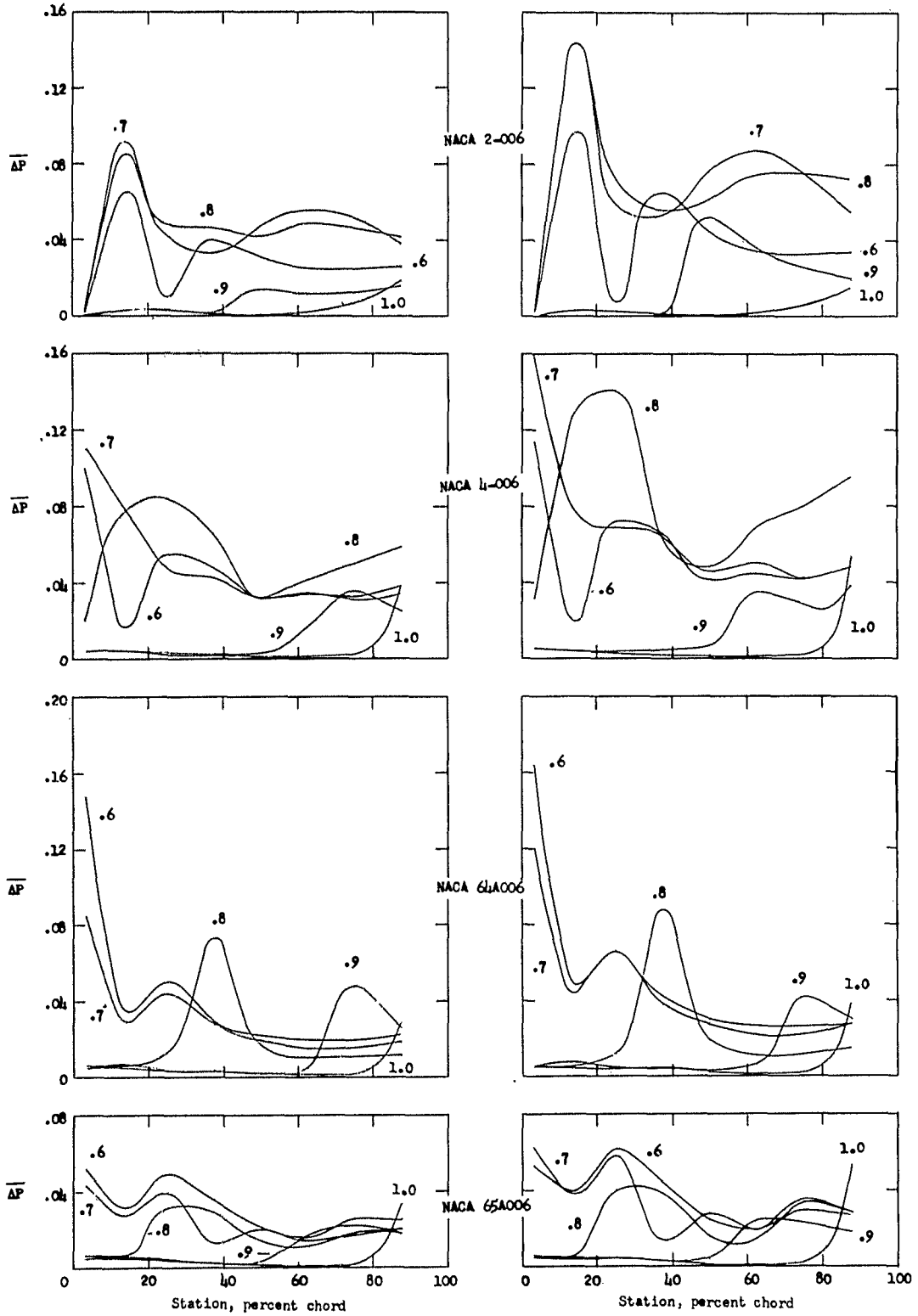
(d) c_n = 0.675 .
