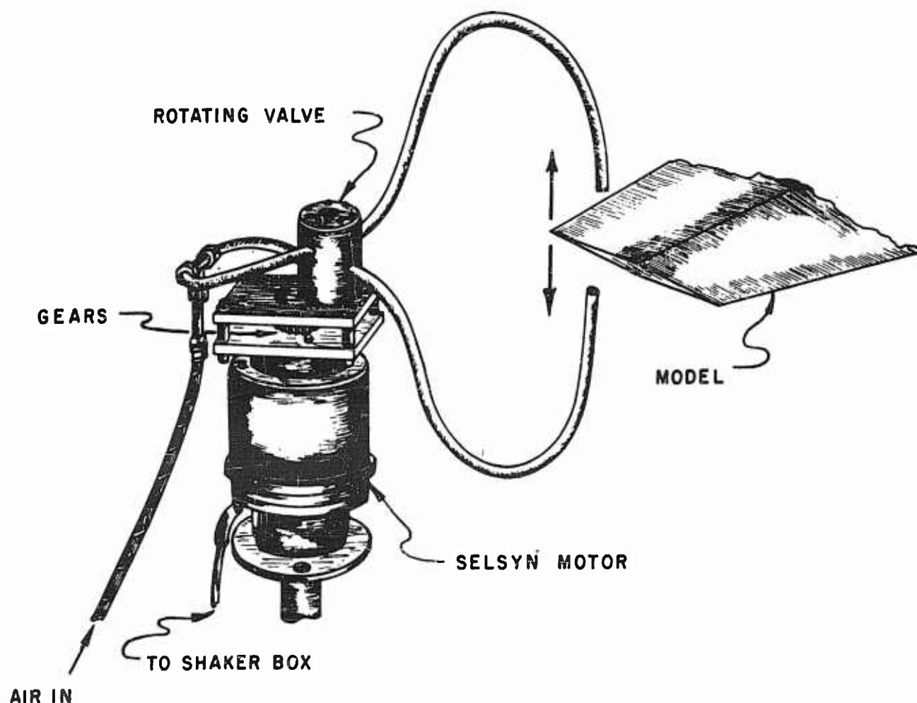
Fig. 18. Air jet shaker unit.
