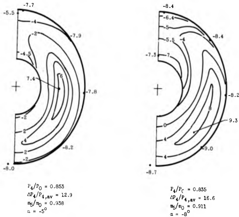
(b) Inlet C_{17S} .
