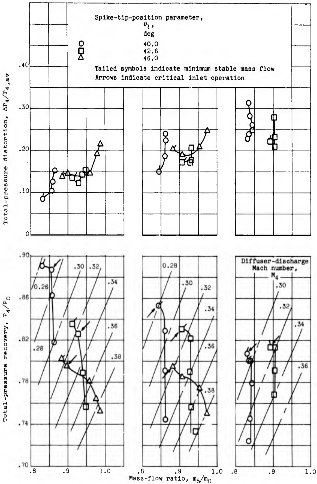
(d) Angle of attack, -3^\circ ; free-stream Mach number, 2.0.
