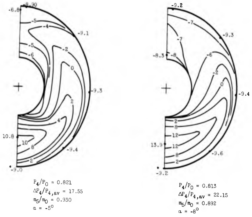
(d) Inlet C_{17S_b} .
