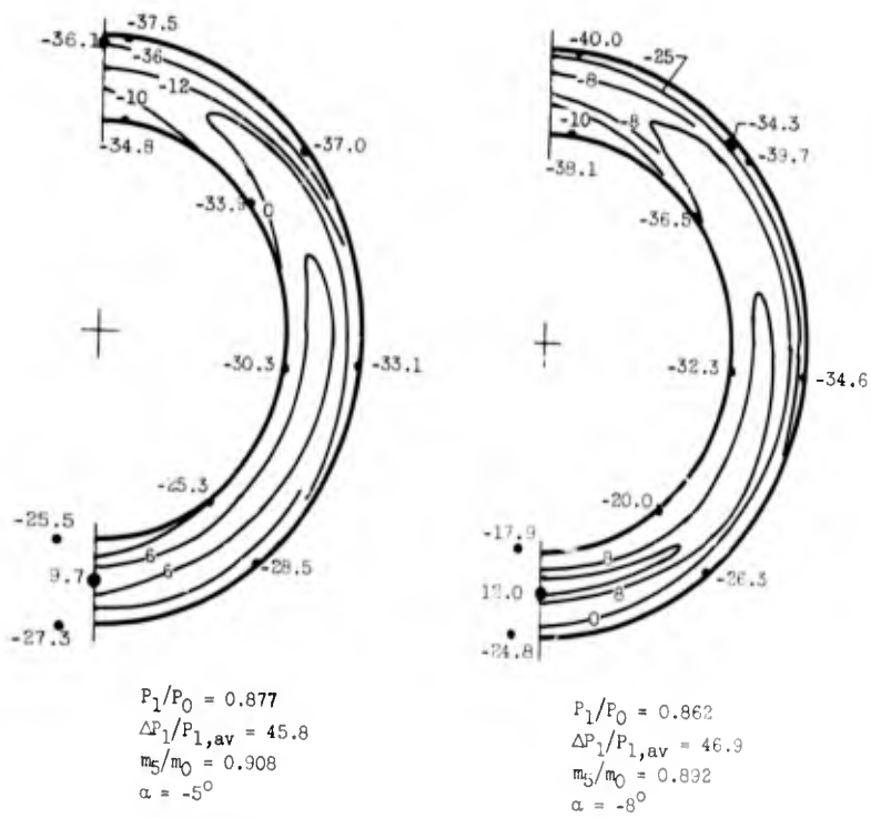
(d) Inlet C_{17S_b} . Spike-tip-position parameter, 42.6^\circ .
