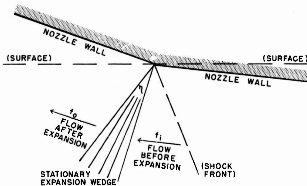
FIG. 2 PRANDTL-MEYER CORNER FLOW
