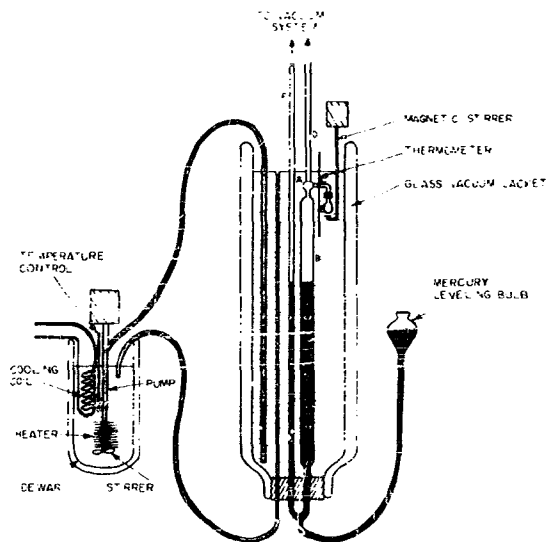
Fig. 9 - Amine resin \text{CO}_2 equilibrium apparatus
