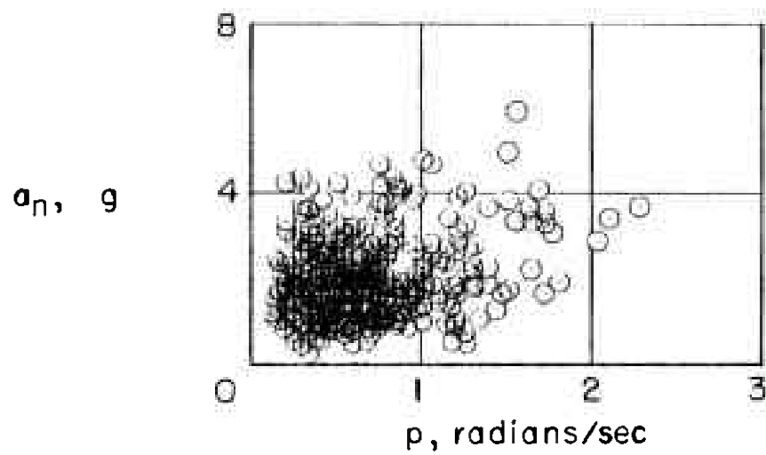
(d) Initial normal acceleration.
