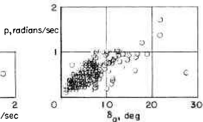
(d) Rolling velocity.
