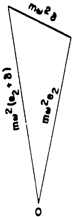
Fig. 15. Force diagram.
