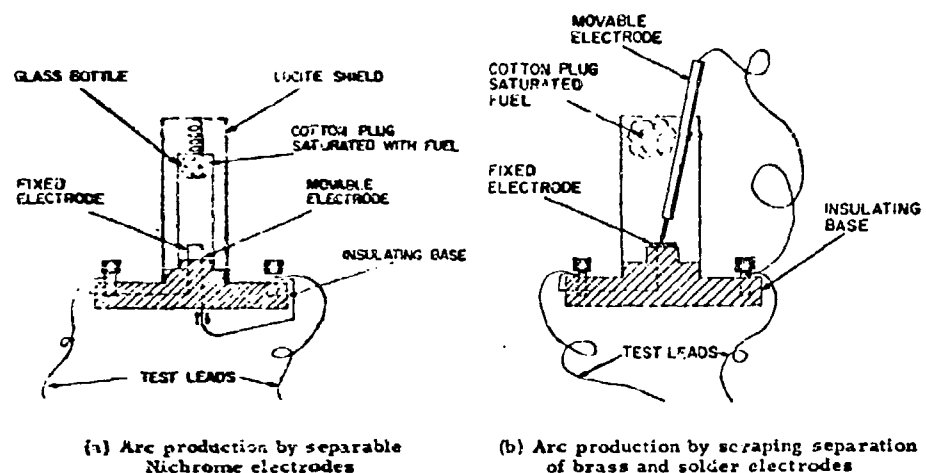
Fig. 1 - Ignition test apparatus
