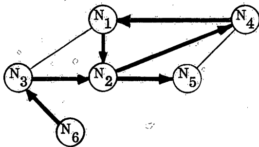
b. An N_6/N_5 path
