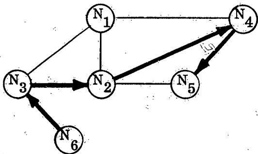
d. N_6/N_5 chain
