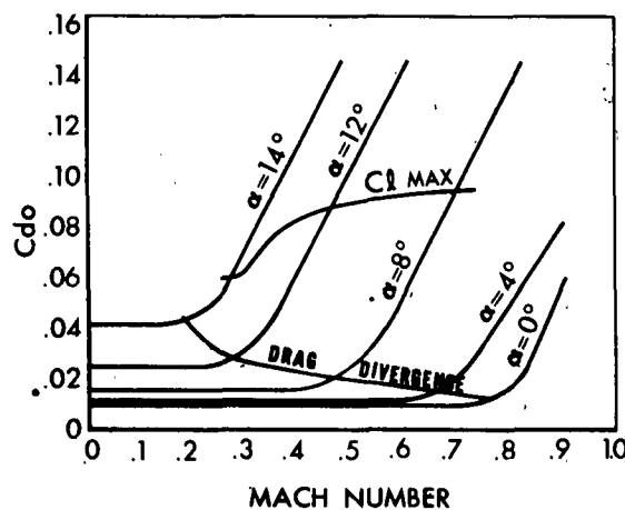
NACA 0012 AIRFOIL
