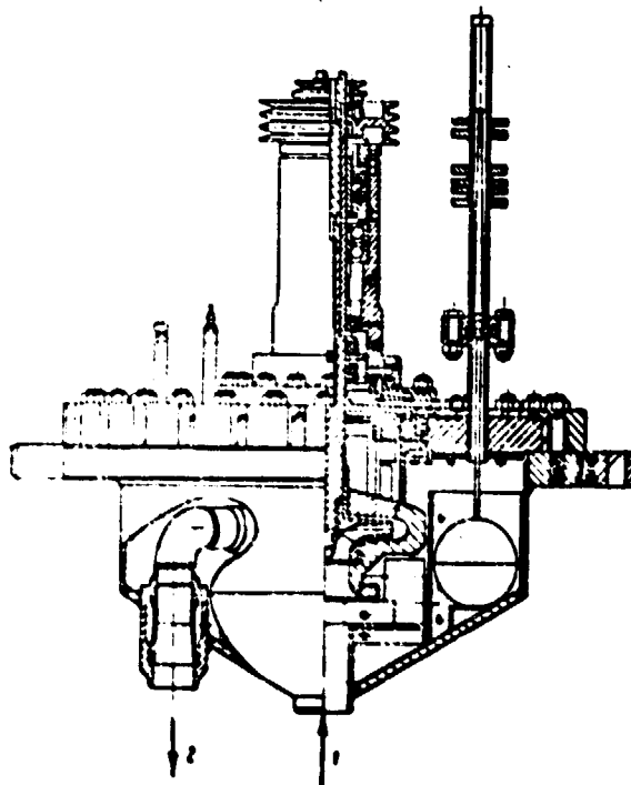
Рис. 130 Центробежный насос с торцевым газонепроницаемым уплотнением
