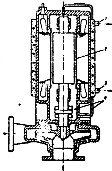
Рис. 125. Насос с разрывом диафрагмы порочен
