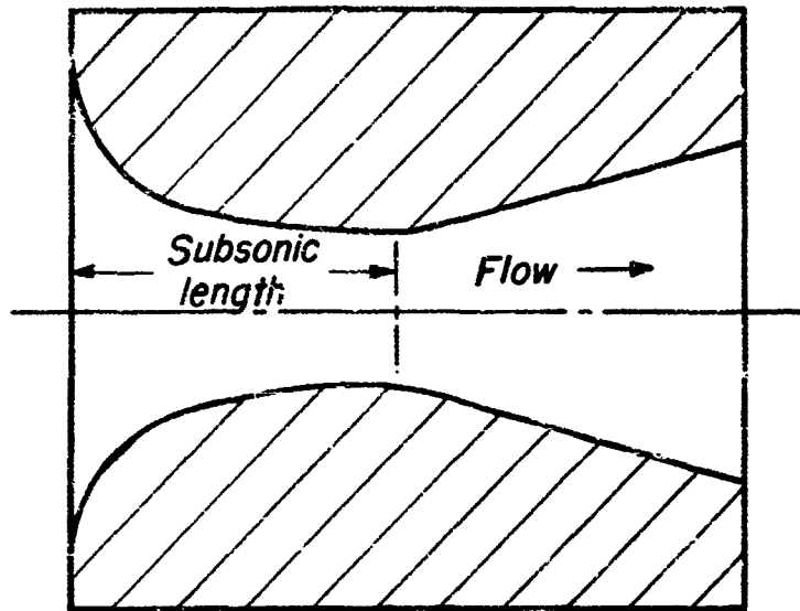
Linear nozzle
