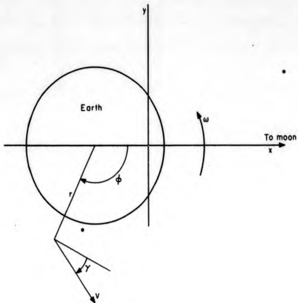
Fig.2—Initial trajectory parameters
