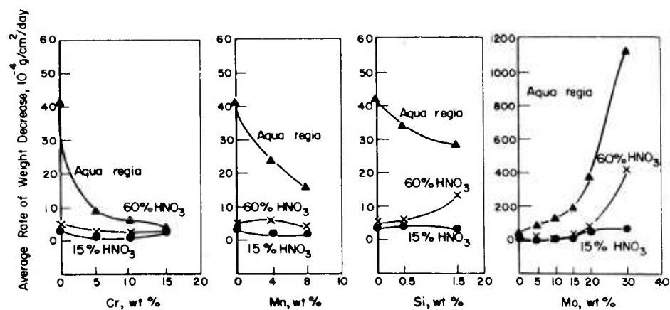
c. In HNO 3 and Aqua Regia at Boiling Temperature
