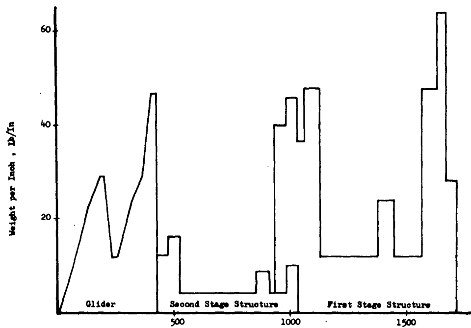
FIG. A-2 WEIGHT EMPTY
