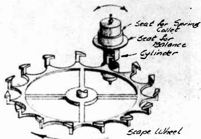
CYLINDER ESCAPEMENT
