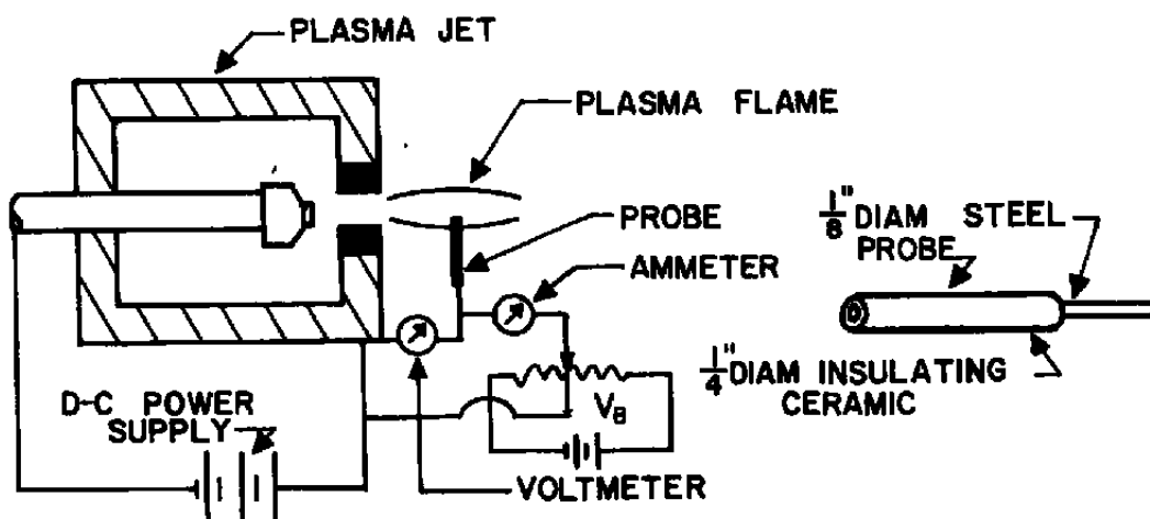
SCHEMATIC VI
