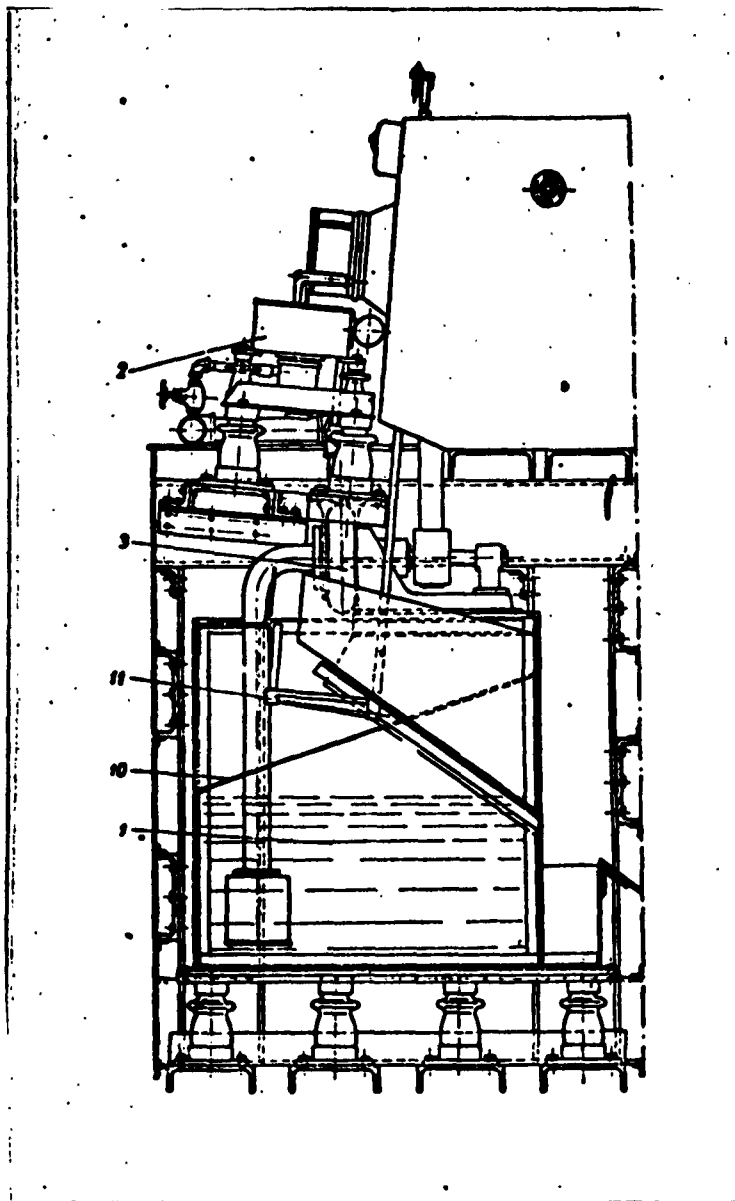
Fig. 73. Automat AE - 9
