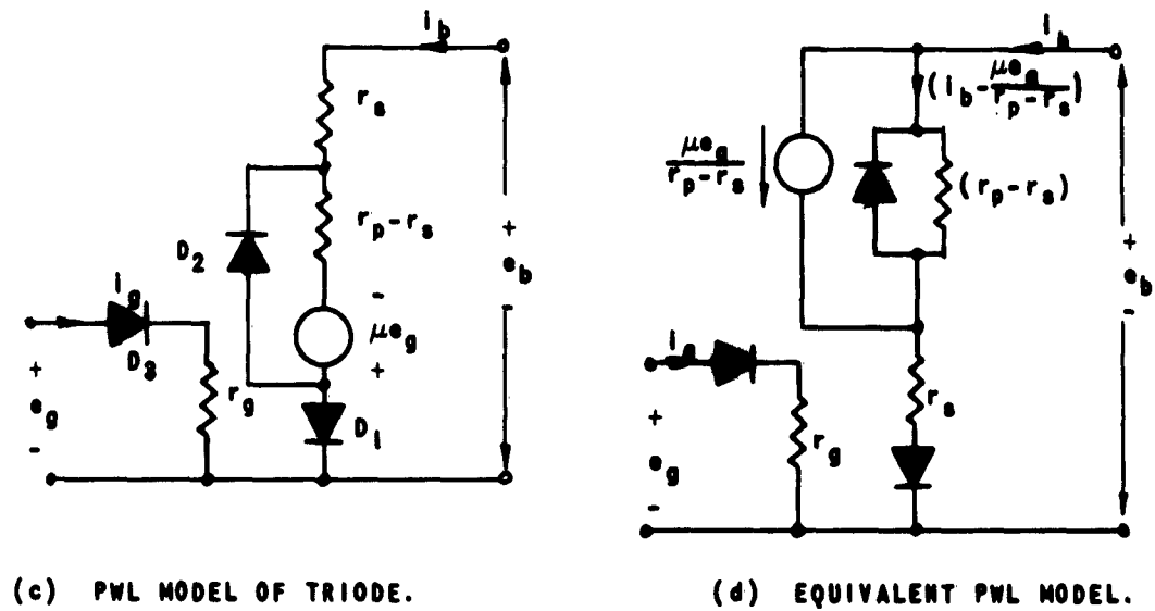
FIG. 50. PWL TRIODE.
