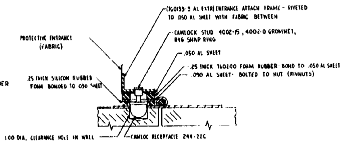
SECTION C-C SCALE: 1/2
