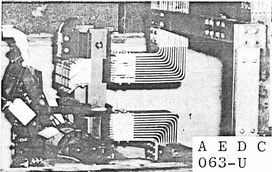
Fig. 22 Breaker
