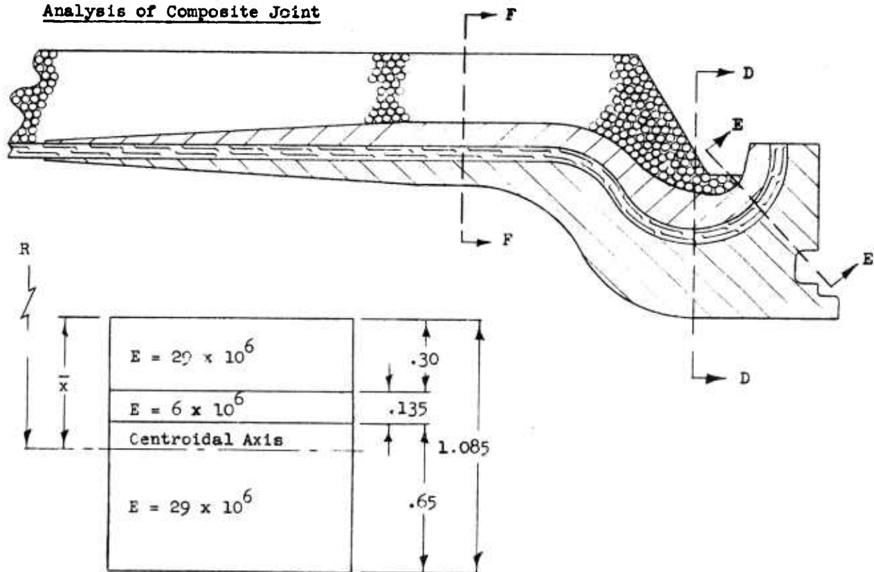
Section D-D
