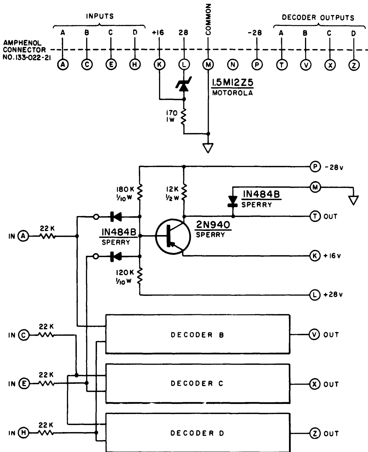
FIG. A-15 DECODER CIRCUITS
