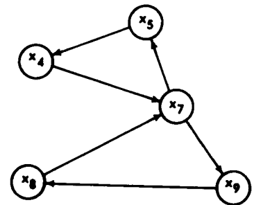
d. A cycle
