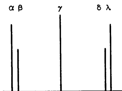
Fig. 17. Mn^{++} ESR due to a given m.
