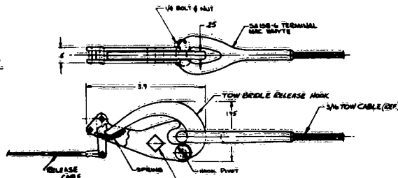
DETAIL B SCALE: 1/4
