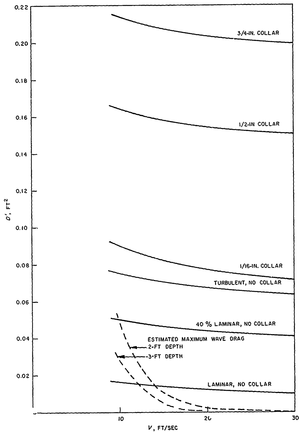
FIG. 5. Drag-Area Estimates.
