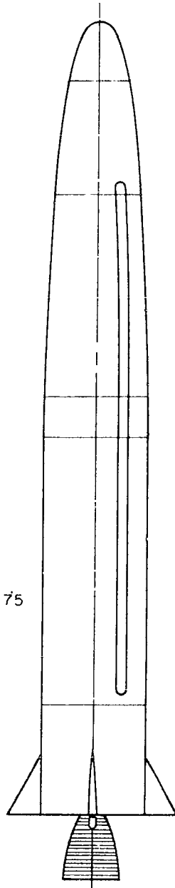
Fig. F-1—General arrangement
